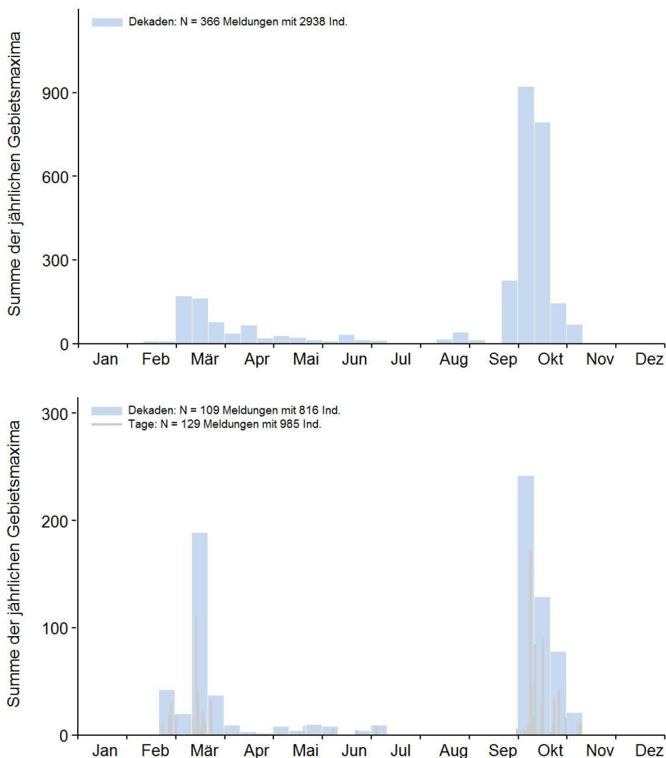
Phänologie der Heideelerche in der Region Neckar-Alb 2010-2015 (oben) sowie 2016 (unten).
