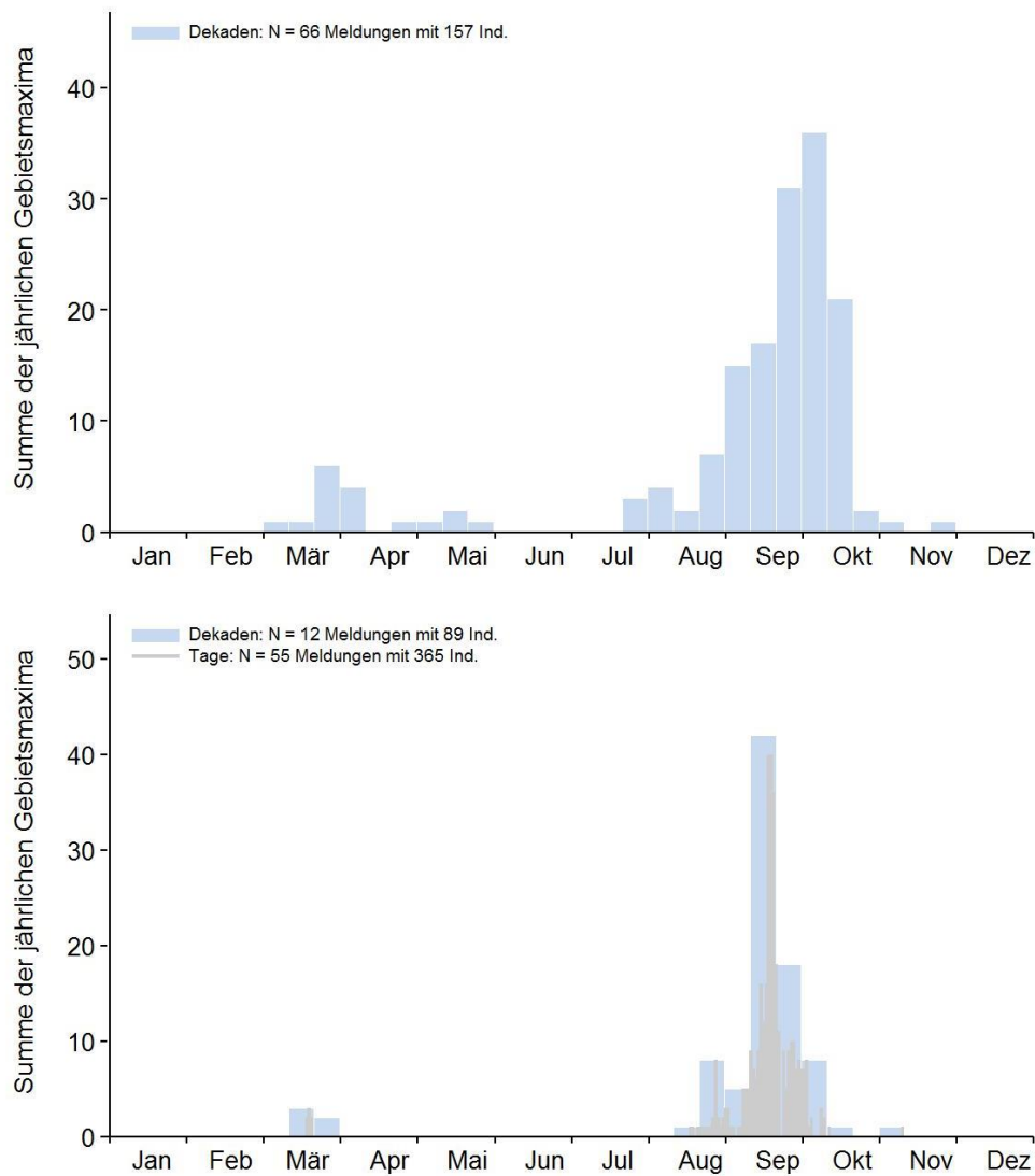
Phänologie des Alpenstrandläufers in der Region Neckar-Alb 2010-2015 (oben) sowie 2016 (unten).
