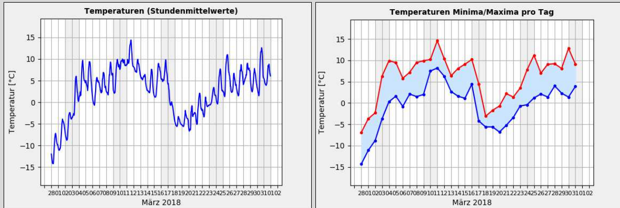
Gr. 1: Temperaturmittelwerte pro Std. in °C vom 01.03. - 31.03.2018; Quelle: Wetterstation der Sternwarte "Welzheim"*
