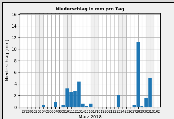
Gr. 3: Niederschlagssumme in mm pro Tag vom 01.03. - 31.03.2018; Quelle: Wetterstation der Sternwarte "Welzheim"*
