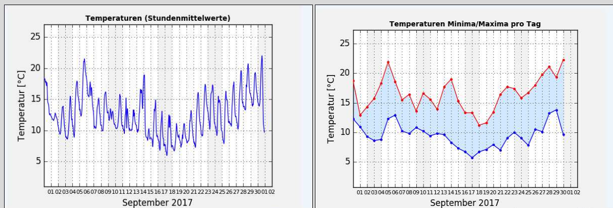
Gr. 1: Temperaturmittelwerte pro Std. in °C vom 01.09. - 30.09.2017; Quelle: Wetterstation der Sternwarte "Welzheim"*
