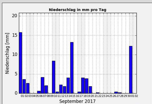
Gr. 3: Niederschlagssumme in mm pro Tag vom 01.09. - 30.09.2017; Quelle: Wetterstation der Sternwarte "Welzheim"*
