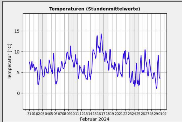
Gr. 1: Temperaturmittelwerte pro Std. in °C vom 01.02. - 29.02.2024; Quelle: Wetterstation der Sternwarte "Welzheim"*
