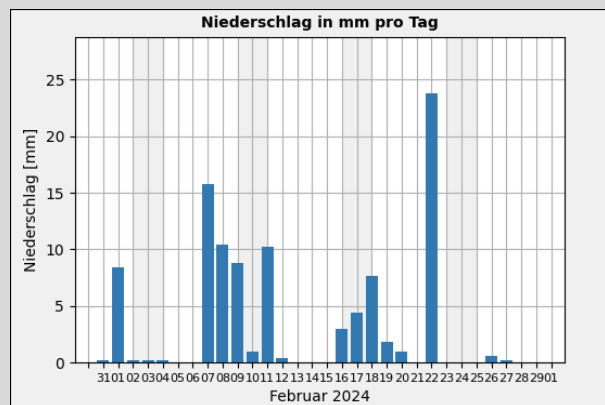
Gr. 3: Niederschlagssumme in mm pro Tag vom 01.02. - 29.02.2024; Quelle: Wetterstation der Sternwarte "Welzheim"*
