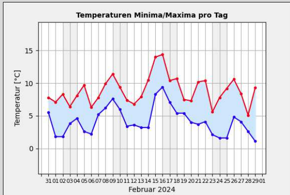
Gr. 2: Temperaturhöchst- u. -tiefstwerte pro Tag in °C vom 01.02. - 29.02.2024; Quelle: Wetterstation der Sternwarte "Welzheim"*
