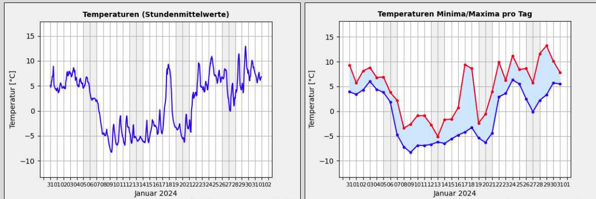
Gr. 1: Temperaturmittelwerte pro Std. in °C vom 01.01. - 31.01.2024; Quelle: Wetterstation der Sternwarte "Welzheim"*
