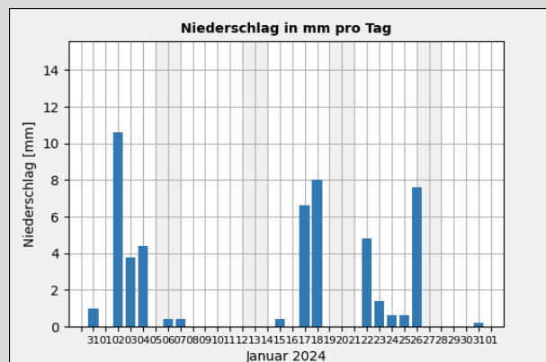
Gr. 3: Niederschlagssumme in mm pro Tag vom 01.01. - 31.01.2024; Quelle: Wetterstation der Sternwarte "Welzheim"*
