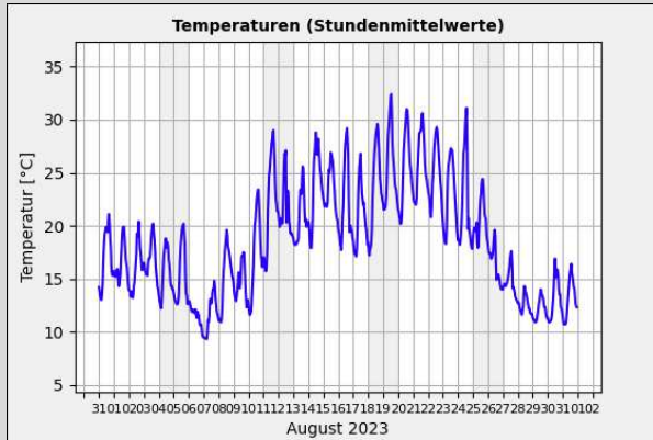
Gr. 1: Temperaturmittelwerte pro Std. in °C vom 01.08. - 31.08.2023; Quelle: Wetterstation der Sternwarte "Welzheim"*
