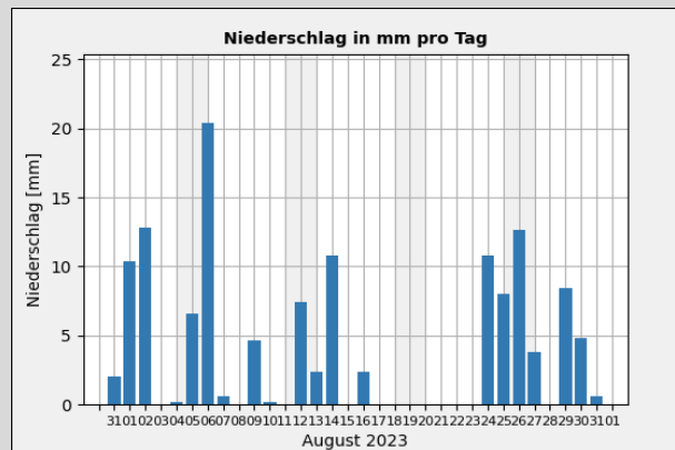
Gr. 3: Niederschlagssumme in mm pro Tag vom 01.08. - 31.08.2023; Quelle: Wetterstation der Sternwarte "Welzheim"*
