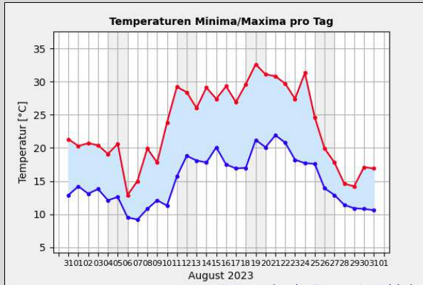
Gr. 2: Temperaturhöchst- u. -tiefstwerte pro Tag in °C vom 01.08. - 31.08.2023; Quelle: Wetterstation der Sternwarte "Welzheim"*
