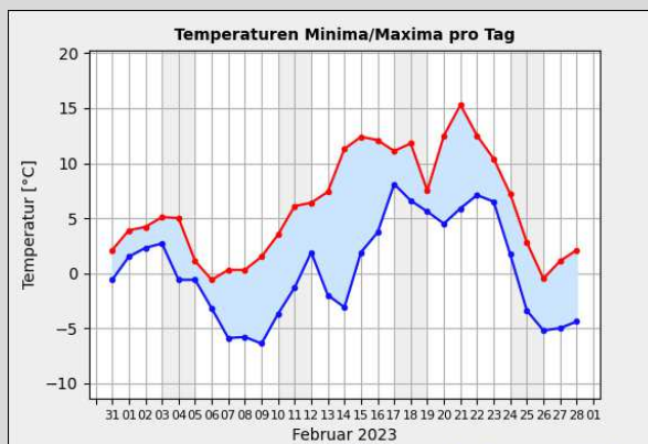
Gr. 2: Temperaturhöchst- u. -tiefstwerte pro Tag in °C vom 01.02. - 28.02.2023; Quelle: Wetterstation der Sternwarte "Welzheim"*
