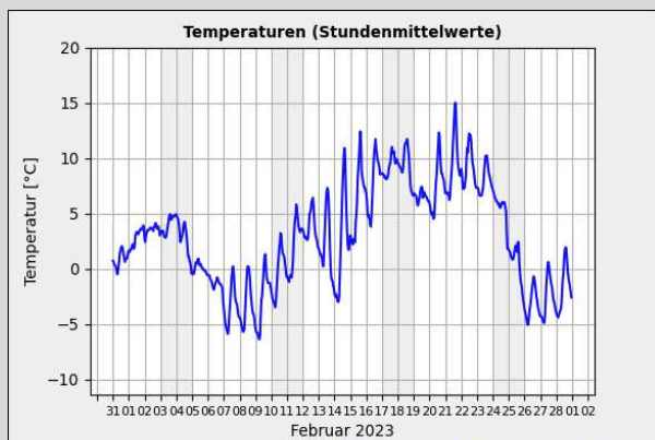
Gr. 1: Temperaturmittelwerte pro Std. in °C vom 01.02. - 28.02.2023; Quelle: Wetterstation der Sternwarte "Welzheim"*
