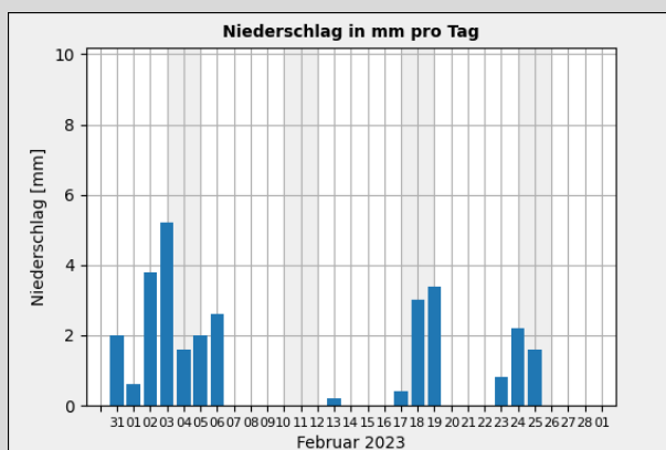
Gr. 3: Niederschlagssumme in mm pro Tag vom 01.02. - 28.02.2023; Quelle: Wetterstation der Sternwarte "Welzheim"*
