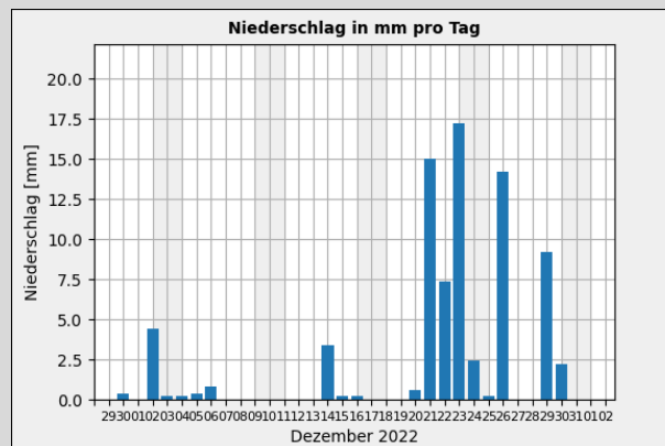
Gr. 3: Niederschlagssumme in mm pro Tag vom 01.12. - 31.12.2022; Quelle: Wetterstation der Sternwarte "Welzheim"*
