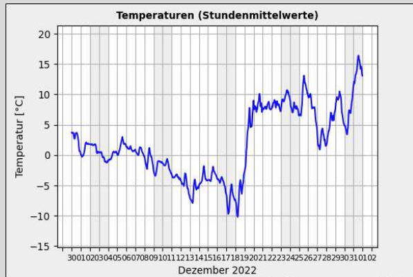
Gr. 1: Temperaturmittelwerte pro Std. in °C vom 01.12. - 31.12.2022; Quelle: Wetterstation der Sternwarte "Welzheim"*
