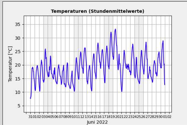
Gr. 1: Temperaturmittelwerte pro Std. in °C vom 01.06. - 30.06.2022; Quelle: Wetterstation der Sternwarte "Welzheim"*
