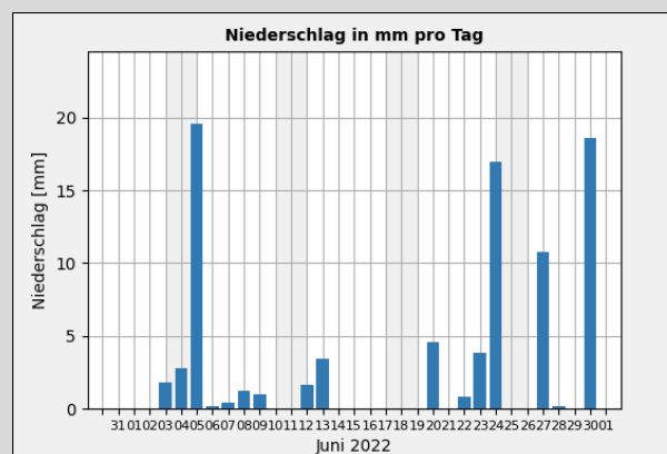
Gr. 3: Niederschlagssumme in mm pro Tag vom 01.06. - 30.06.2022; Quelle: Wetterstation der Sternwarte "Welzheim"*
