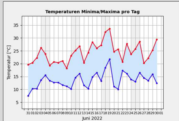
Gr. 2: Temperaturhöchst- u. -tiefstwerte pro Tag in °C vom 01.06. - 30.06.2022; Quelle: Wetterstation der Sternwarte "Welzheim"*
