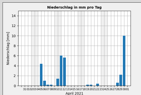
Gr. 3: Niederschlagssumme in mm pro Tag vom 01.04. - 30.04.2021; Quelle: Wetterstation der Sternwarte "Welzheim"*
