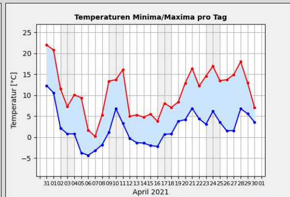
Gr. 2: Temperaturhöchst- u. -tiefstwerte pro Tag in °C vom 01.04. - 30.04.2021; Quelle: Wetterstation der Sternwarte "Welzheim"*
