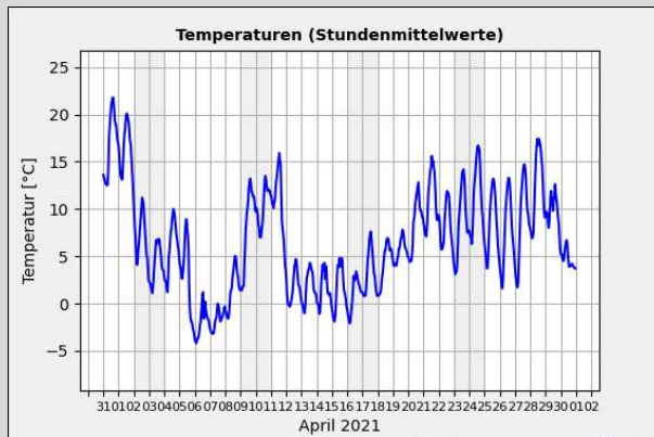
Gr. 1: Temperaturmittelwerte pro Std. in °C vom 01.04. - 30.04.2021; Quelle: Wetterstation der Sternwarte "Welzheim"*
