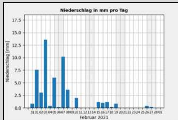
Gr. 3: Niederschlagssumme in mm pro Tag vom 01.02. - 28.02.2021; Quelle: Wetterstation der Sternwarte "Welzheim"*
