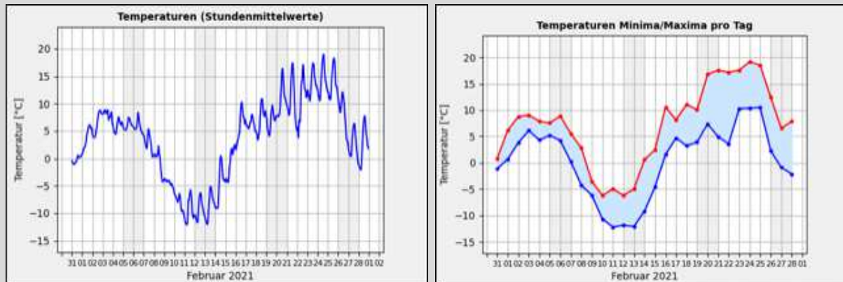
Gr. 1: Temperaturmittelwerte pro Std. in °C vom 01.02. - 28.02.2021; Quelle: Wetterstation der Sternwarte "Welzheim"*
