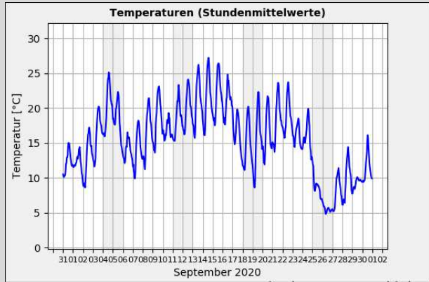
Gr. 1: Temperaturmittelwerte pro Std. in °C vom 01.09. - 30.09.2020; Quelle: Wetterstation der Sternwarte "Welzheim"*
