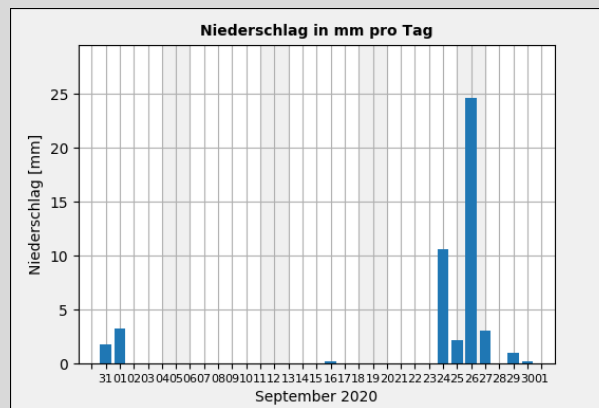
Gr. 3: Niederschlagssumme in mm pro Tag vom 01.09. - 30.09.2020; Quelle: Wetterstation der Sternwarte "Welzheim"*
