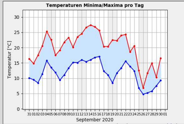
Gr. 2: Temperaturhöchst- u. -tiefstwerte pro Tag in °C vom 01.09. - 30.09.2020; Quelle: Wetterstation der Sternwarte "Welzheim"*
