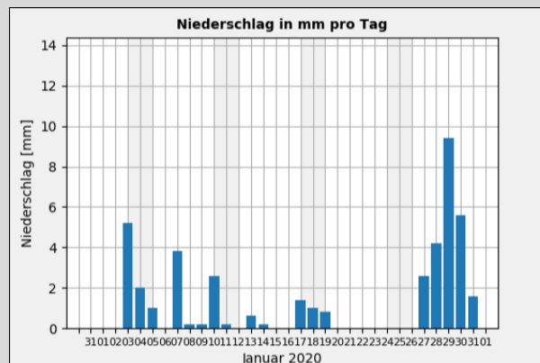
Gr. 3: Niederschlagssumme in mm pro Tag vom 01.01. - 31.01.2020; Quelle: Wetterstation der Sternwarte "Welzheim"*
