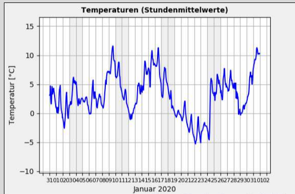
Gr. 1: Temperaturmittelwerte pro Std. in °C vom 01.01. - 31.01.2020; Quelle: Wetterstation der Sternwarte "Welzheim"*
