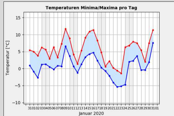
Gr. 2: Temperaturhöchst- u. -tiefstwerte pro Tag in °C vom 01.01. - 31.01.2020; Quelle: Wetterstation der Sternwarte "Welzheim"*
