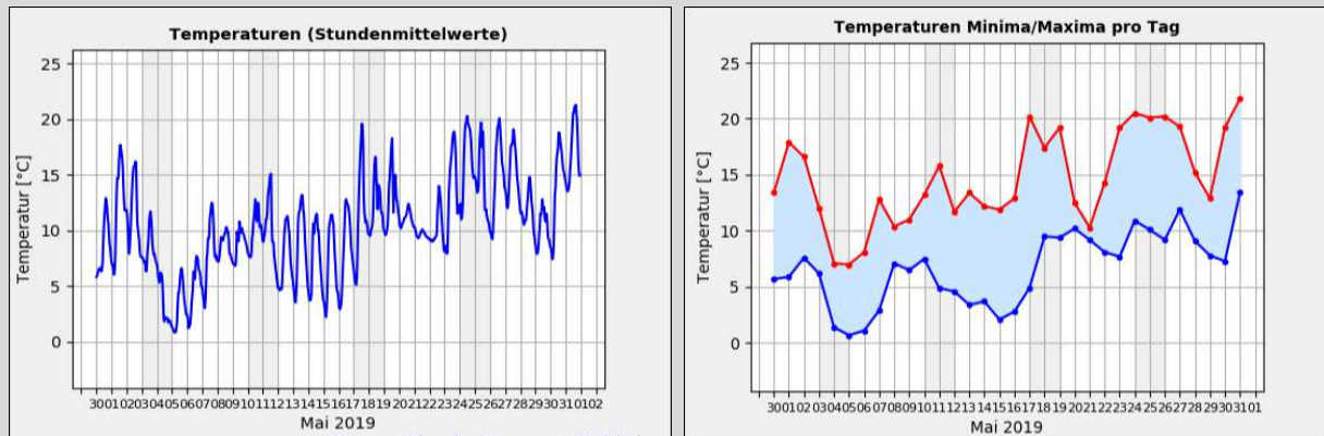
Gr. 1: Temperaturmittelwerte pro Std. in °C vom 01.05. - 31.05.2019; Quelle: Wetterstation der Sternwarte "Welzheim"*
