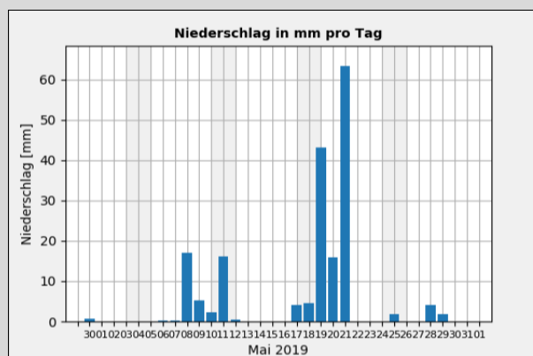
Gr. 3: Niederschlagssumme in mm pro Tag vom 01.05. - 31.05.2019; Quelle: Wetterstation der Sternwarte "Welzheim"*
