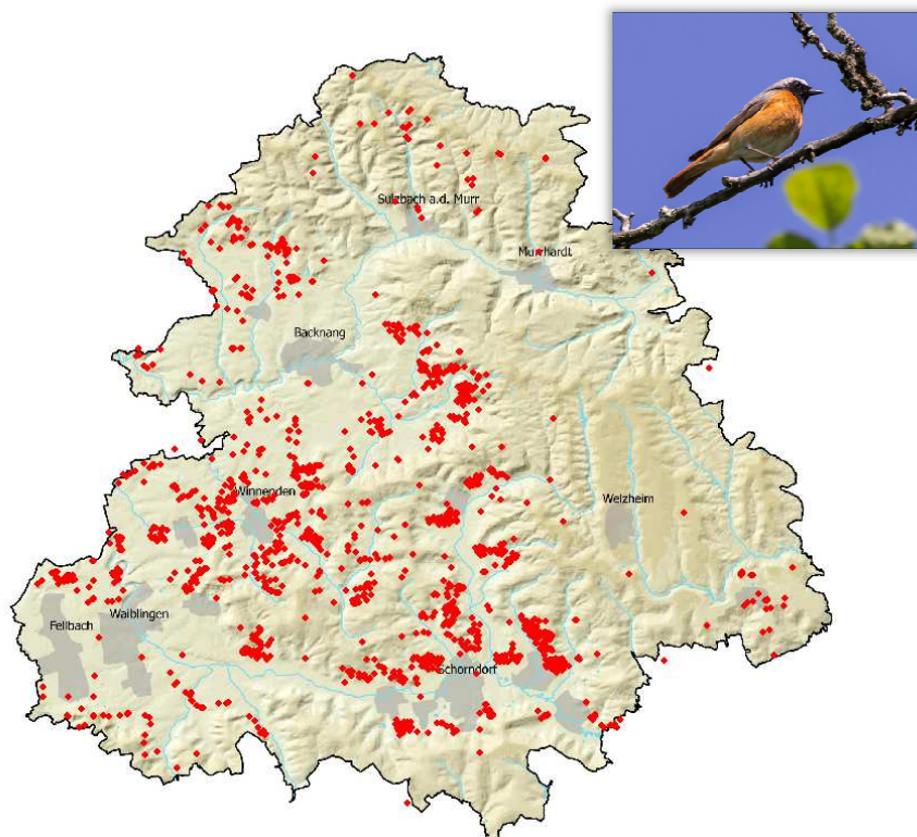
Abb. 2: Kartographische Darstellung aller gemeldeten Mai-Beobachtungen der Jahre 2015 - 2019 (n = 1.758 Beob.) des Gartenrotschwanzes Phoenicurus phoenicurus aus dem Kreisgebiet Rems-Murr. Durch das umfangreiche Datenmaterial der zurückliegenden Jahre lässt sich ein aussagekräftiges Bild der kreisweiten Brutverbreitung der Art gewinnen. Beachten Sie bitte, dass die Darstellung auch Gebietsverortungen und Mehrfachmeldungen enthält. Foto: 1.0 ad. Ind. Gartenrotschwanzes Phoenicurus phoenicurus Datum: 30.05.2019; Ort: Steinbach; Photograph/in: K. Dahl
