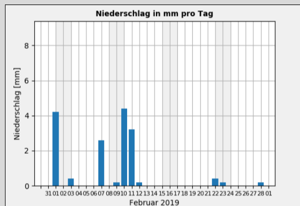
Gr. 3: Niederschlagssumme in mm pro Tag vom 01.02. - 28.02.2019; Quelle: Wetterstation der Sternwarte "Welzheim"*
