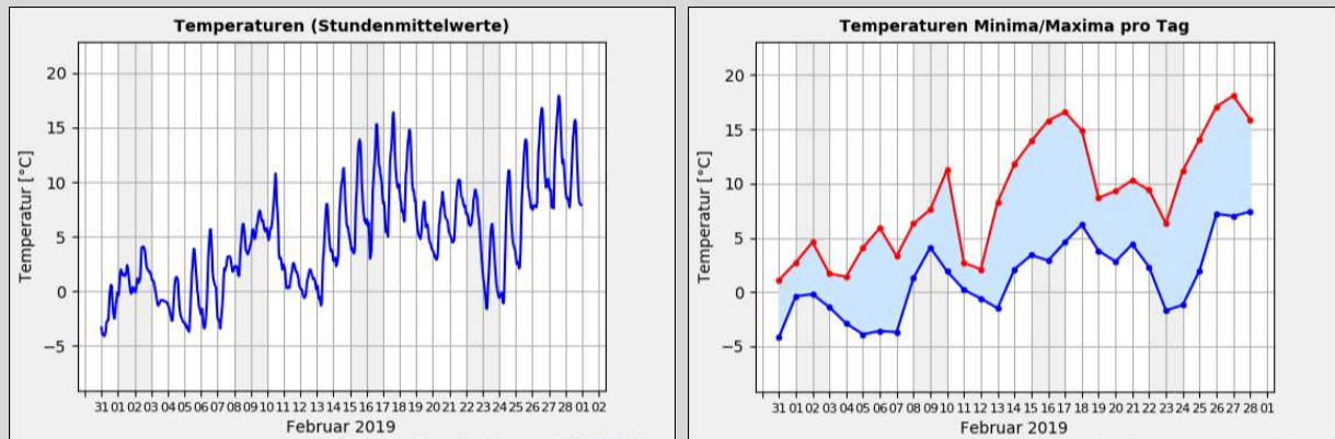
Gr. 1: Temperaturmittelwerte pro Std. in °C vom 01.02. - 28.02.2019; Quelle: Wetterstation der Sternwarte "Welzheim"*
