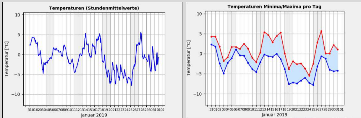
Gr. 1: Temperaturmittelwerte pro Std. in °C vom 01.01. - 31.01.2019; Quelle: Wetterstation der Sternwarte "Welzheim"*
