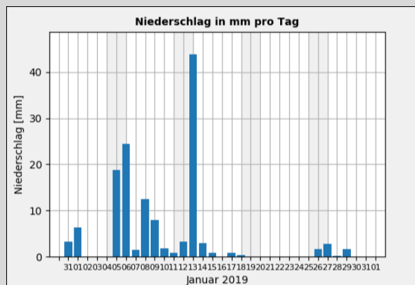
Gr. 3: Niederschlagssumme in mm pro Tag vom 01.01. - 31.01.2019; Quelle: Wetterstation der Sternwarte "Welzheim"*
