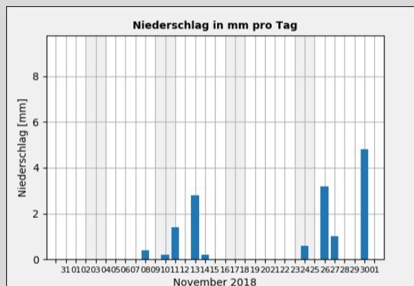
Gr. 3: Niederschlagssumme in mm pro Tag vom 01.11. - 30.11.2018; Quelle: Wetterstation der Sternwarte "Welzheim"*
