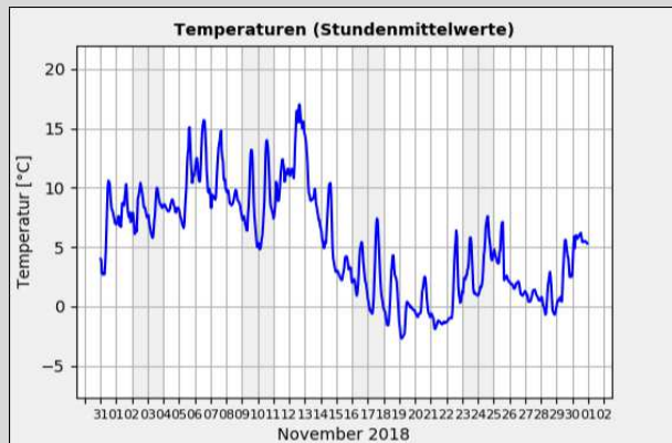
Gr. 1: Temperaturmittelwerte pro Std. in °C vom 01.11. - 30.11.2018; Quelle: Wetterstation der Sternwarte "Welzheim"*
