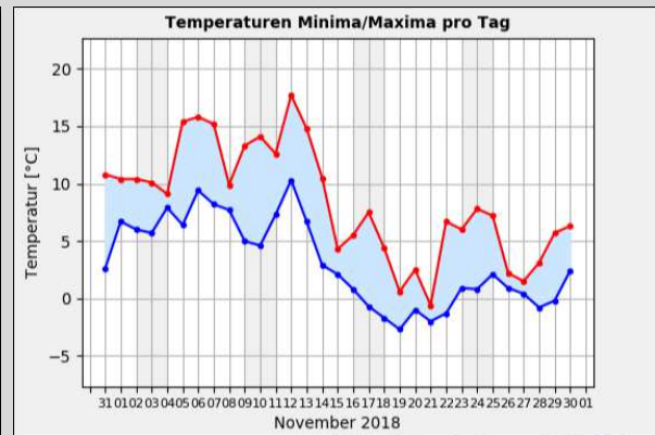
Gr. 2: Temperaturhöchst- u. -tiefstwerte pro Tag in °C vom 01.11. - 30.11.2018; Quelle: Wetterstation der Sternwarte "Welzheim"*
