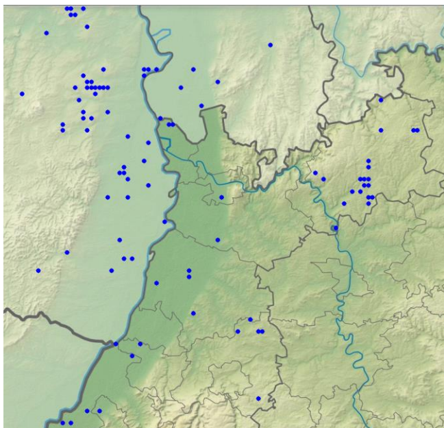
Wachtel-Meldungen 2023
