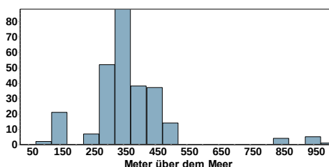
Misteldrossel Höhenverteilung
