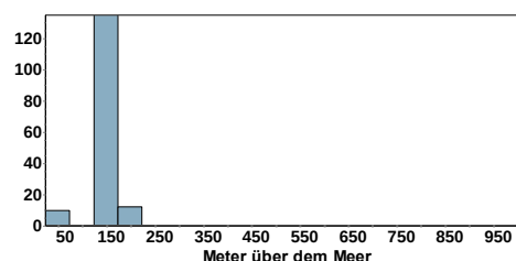
Feldsperling Höhenverteilung
