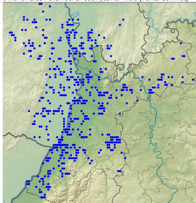
Pirol-Meldungen in 2023
