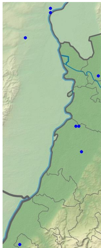
Tüpfelsumpfhuhn-Meldungen in 2023
