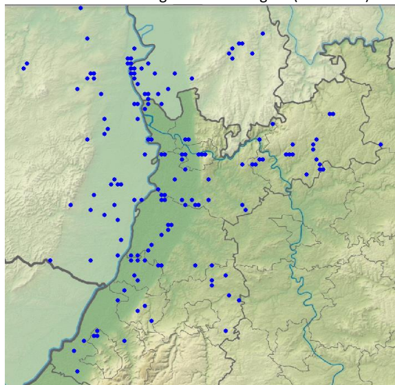
Baumfalken-Meldungen in 2023
