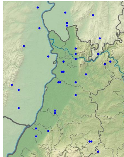
Dohlen-Brutmeldungen (B-Meldungen)
