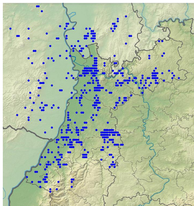
Gartenrotschwanz-Meldungen in 2023
