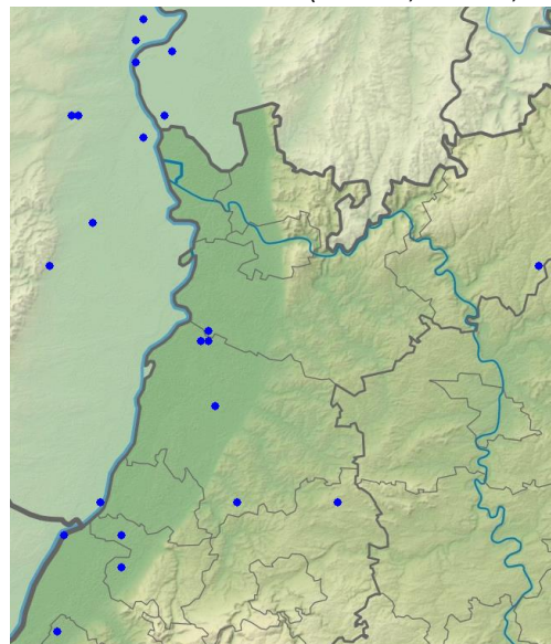
Rotschenkel-Meldungen in 2023
