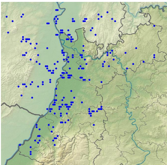
Kleinspecht-Meldungen in 2023
