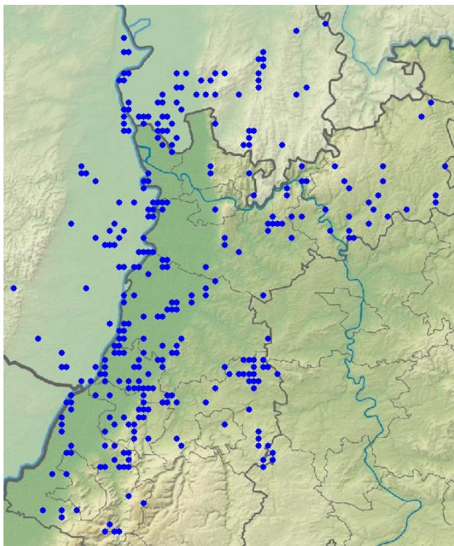
Grünspecht-Meldungen in 2023
