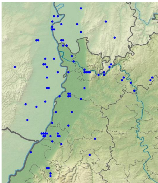
Nilgans-Brutmeldungen (C-Meldungen)
