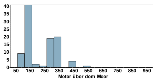
Kernbeißer Höhenverteilung
