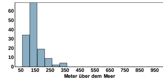
Schwarzkehlchen Höhenverteilung
