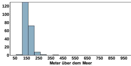
Girlitz Höhenverteilung
