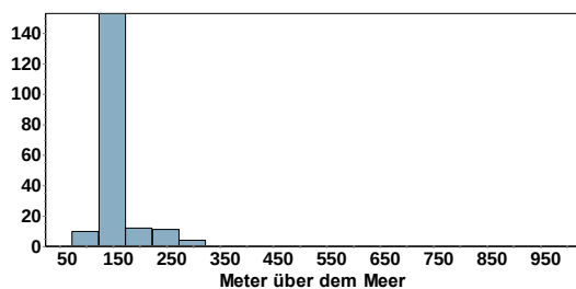
Fasan Höhenverteilung
