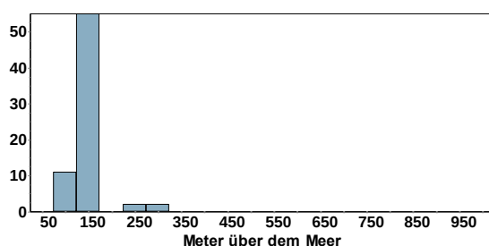
Trauerschnäpper Höhenverteilung
