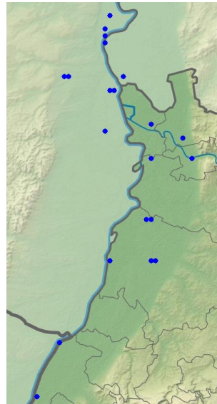
Alpenstrandläufer-Meldungen in 2023
