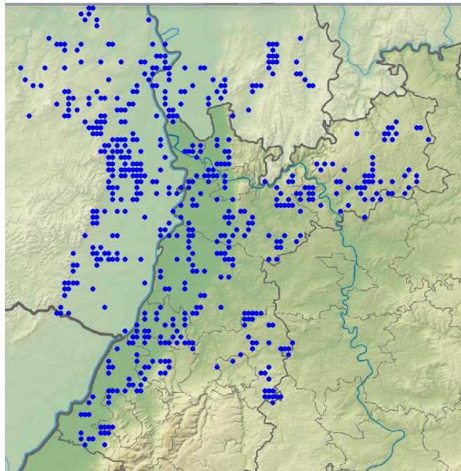
Dorngrasmücken-Meldungen in 2023
