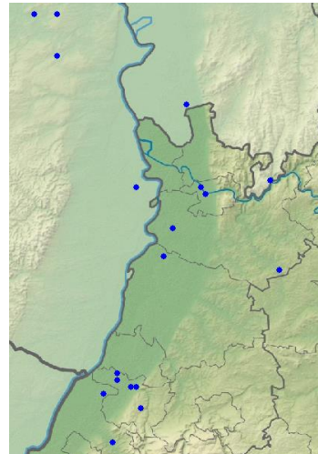
Dohlen-Brutmeldungen (C-Meldungen)
