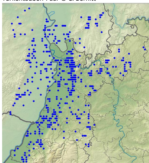
Türkentauben-Meldungen in 2023
