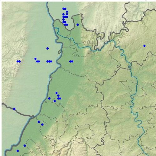
Ziegenmelker-Meldungen in 2023
