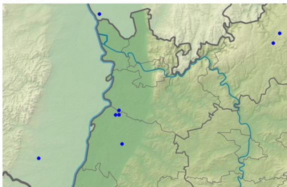
Sichler-Meldungen in 2023
