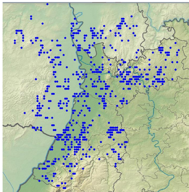
Neuntöter-Meldungen in 2023
