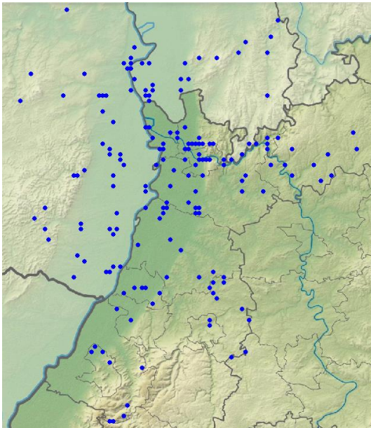
Wanderfalken-Meldungen in 2023
