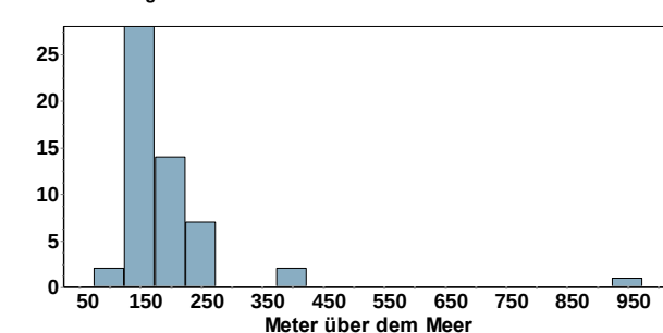
Gartenrotschwanz Höhenverteilung
