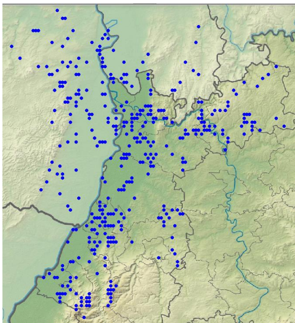
Fitis-Meldungen in 2023
