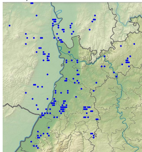
Sumpfrohrsänger-Meldungen in 2023
