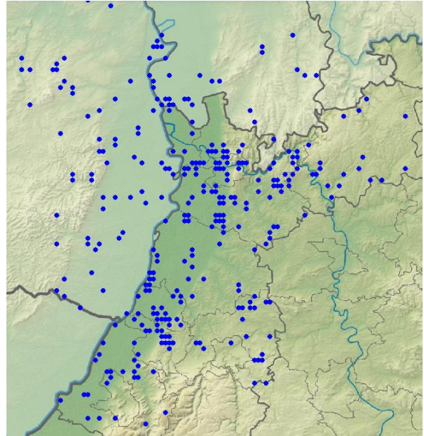
Schwanzmeisen-Meldungen in 2023
