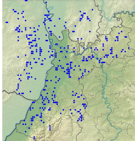
Gartengrasmücken-Meldungen in 2023
