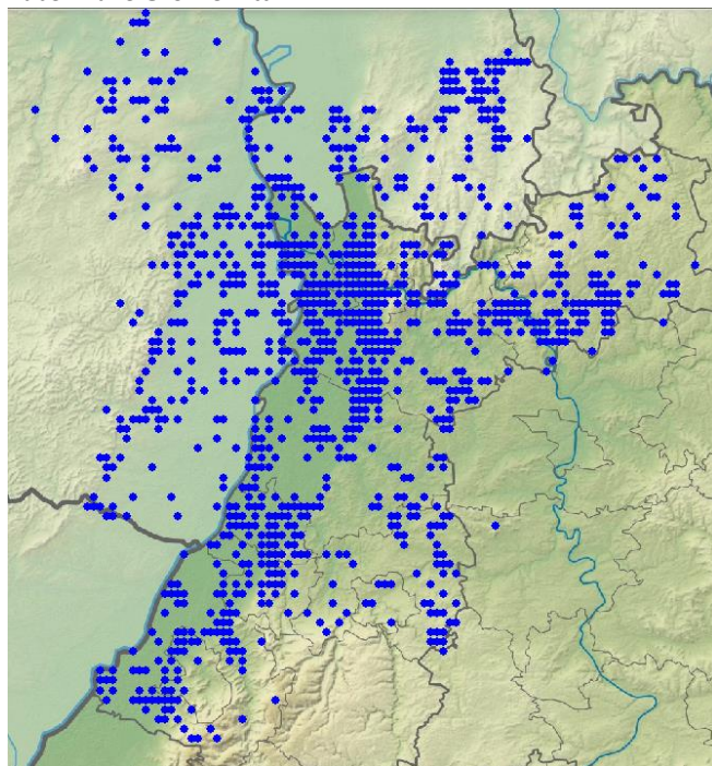
Rabenkrähen-Meldungen in 2023
