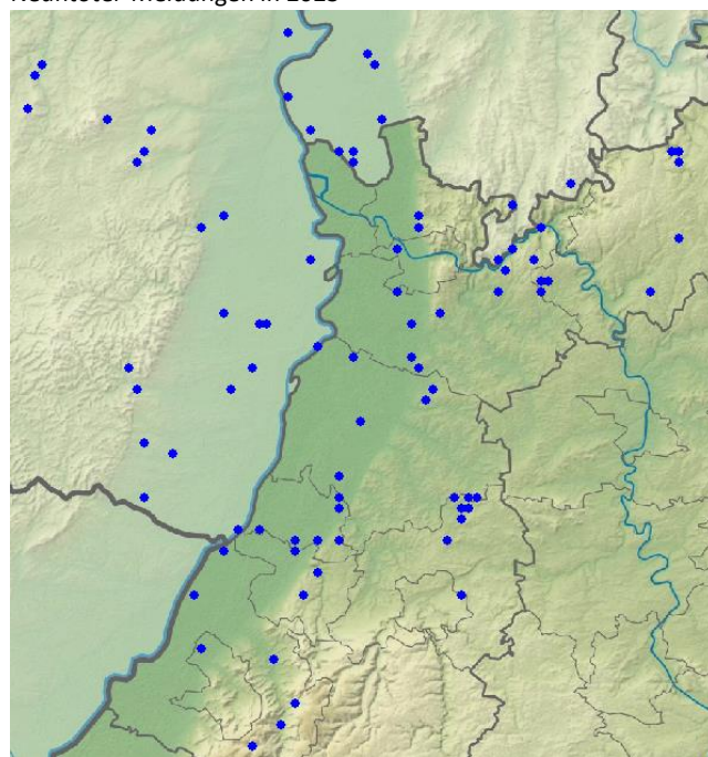
Neuntöter-Brutmeldungen (C-Meldungen)
