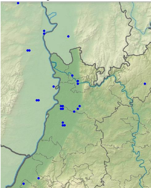
Drosselrohrsänger-Meldungen in 2023
