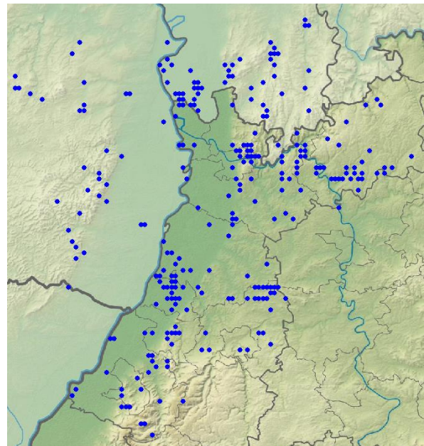
Waldkauz-Meldungen in 2023
