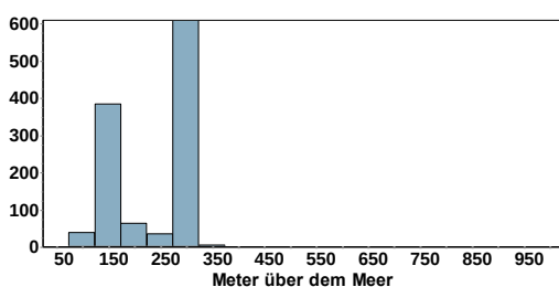
Bluthänfling Höhenverteilung
