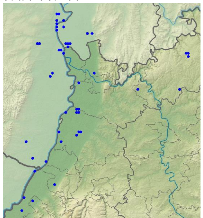
Grünschenkel-Meldungen in 2023
