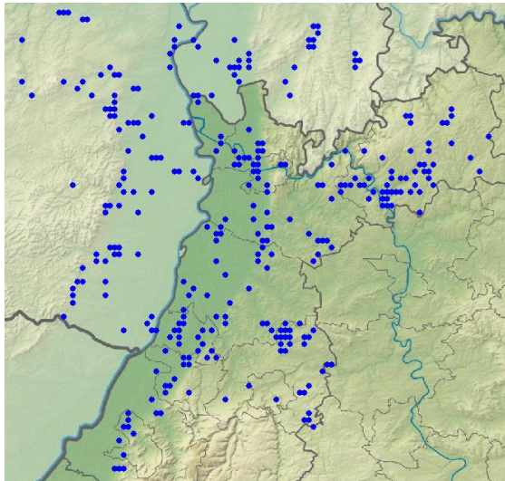
Klappergrasmücken-Meldungen in 2023
