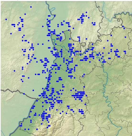
Mittelspecht-Meldungen in 2023
