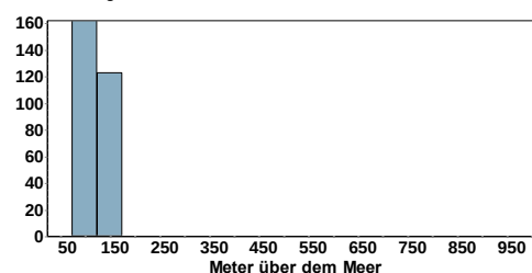
Blaukehlchen Höhenverteilung
